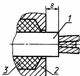
1 - оболочка кабеля; 2 - стенка вводного устройства; 3 - уплотнение Черт. 1
